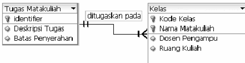
Gambar 2: Hubungan antara Tugas Matakuliah dan entitas baru, Kelas.
